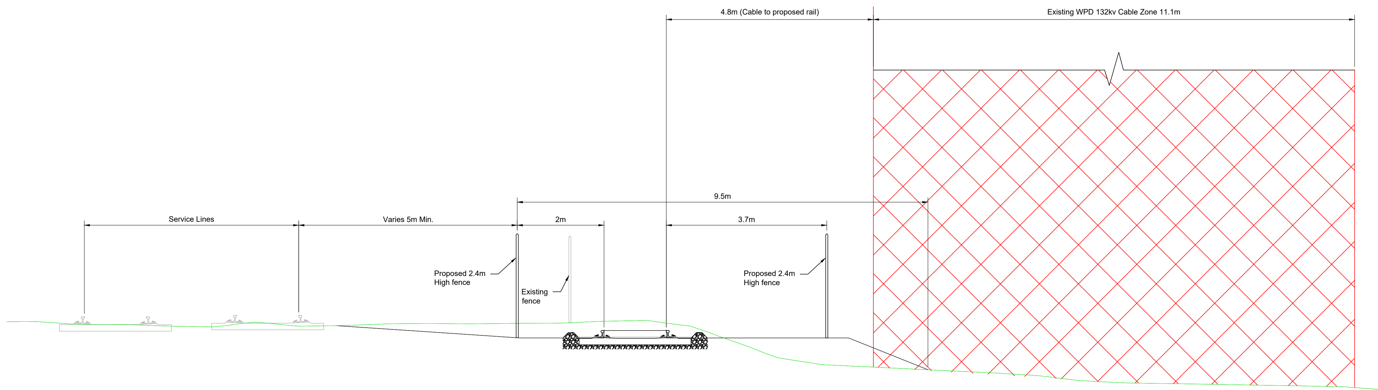
Section B 1:50 0003
