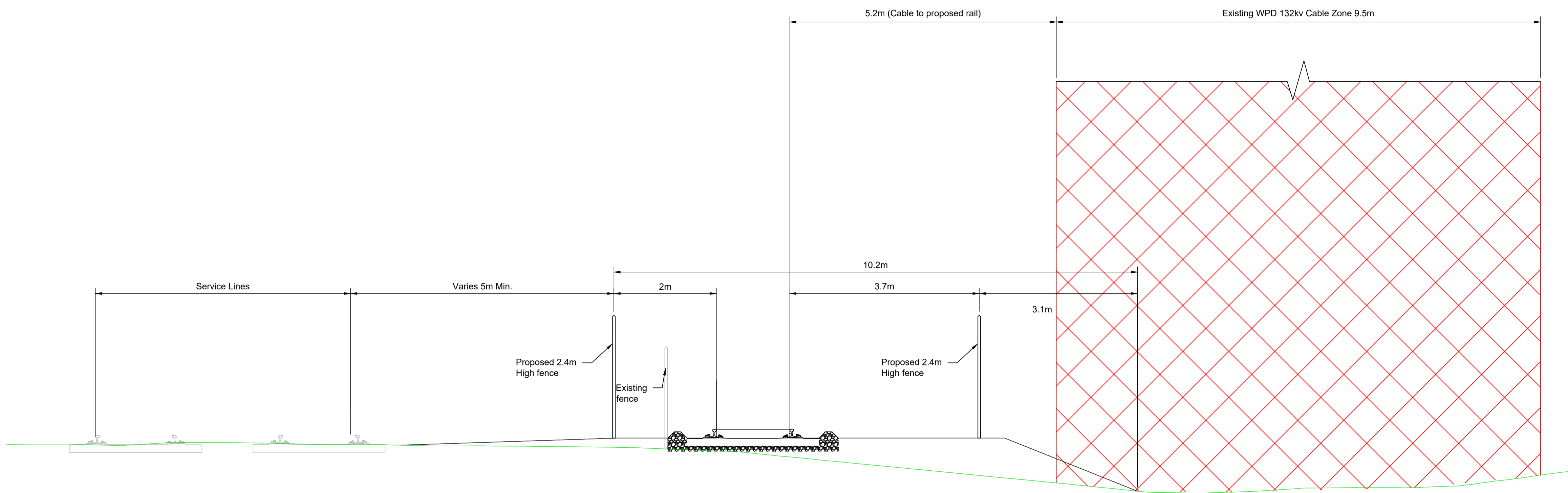
Section A 1:50 0004
